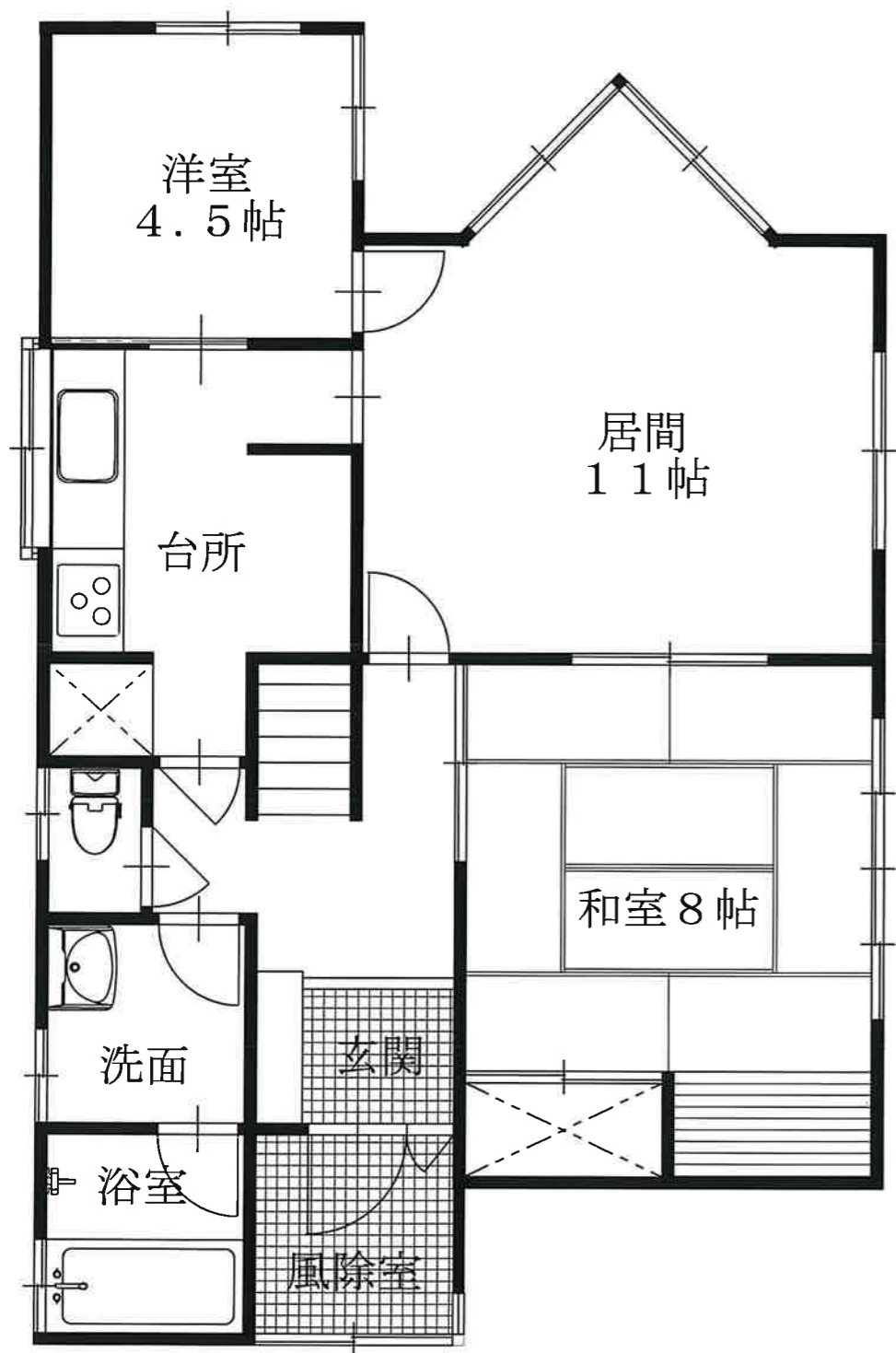
1階平面図
