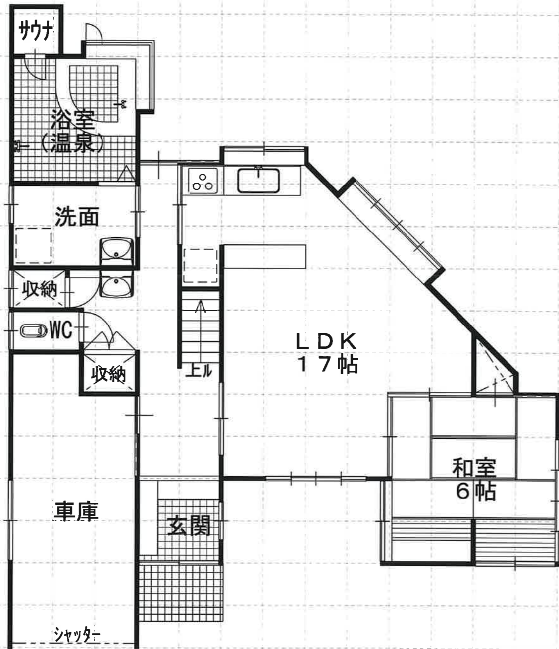
1階平面図
