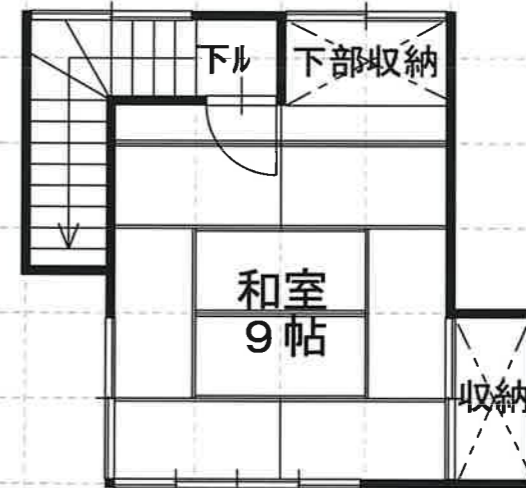
2階平面図
