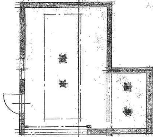
0階平面図
